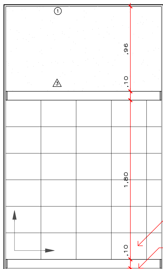
04 EDIFÍCIO ADMINISTRATIVO COPA — EL. 04 AMPLIAÇÕES ESC: ESC: 1:25
