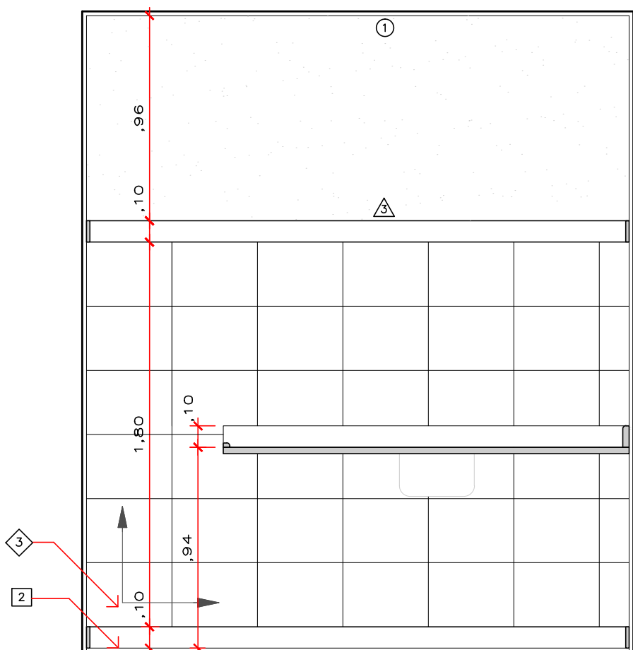
04 EDIFÍCIO ADMINISTRATIVO COPA — EL. 01 AMPLIAÇÕES ESC: ESC: 1:25
