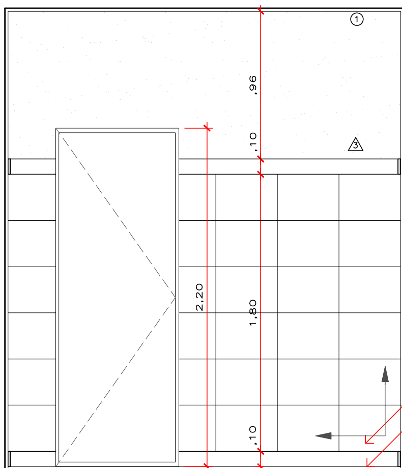
04 EDIFÍCIO ADMINISTRATIVO COPA — EL. 03 AMPLIAÇÕES ESC: ESC: 1:25
